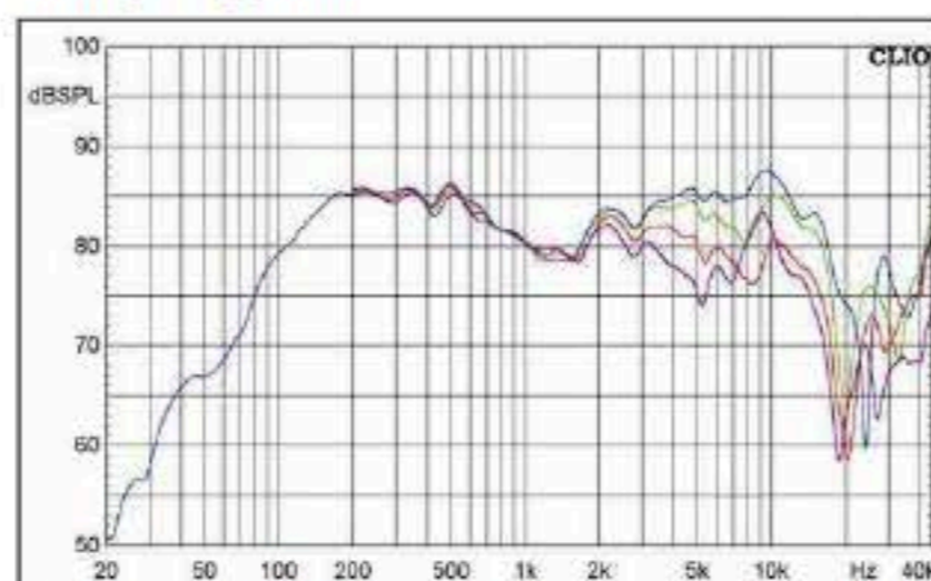
Das Koax-System zeigt eine prima Weichenabstimmung ohne wahrnehmbaren Übergang zwischen Tief- und Hochtöner
