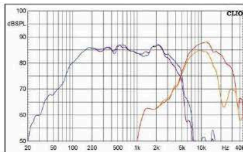
Das Zweiwegensystem trennt bei relativ niedrigen Frequenzen, der 10er-Tieftöner wird besonders wirkungsvoll gefiltert
